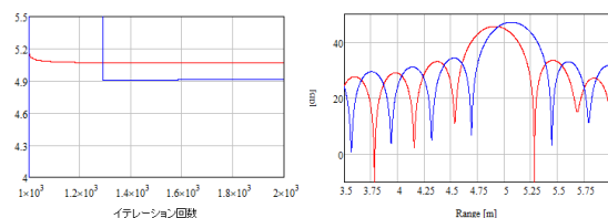
図 1 送信帯域幅 430MHz にて距離分解能 17cm (送信帯域幅と比較して 1/2 の距離分解能) の実験的検証結果
