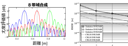
図 5. 離隔周波数コヒーレント合成高分解能化アルゴリズムのシミュレーション評価
