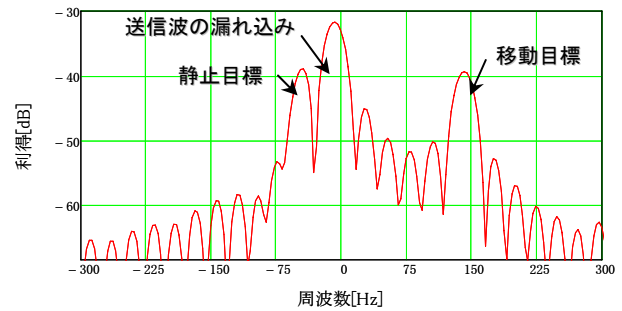
図 2 フーリエ変換の出力結果
