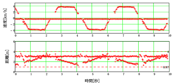
図 3 距離・速度推定結果
