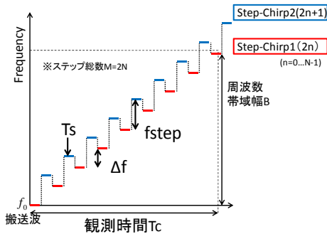
図 1 FMSK 方式の送信シーケンス
