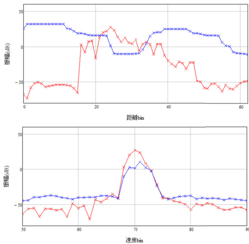
図 6. 目標 1 の速度ビン, 距離ビンにおけるドップラおよびレンジプロファイルと CFAR しきい値
