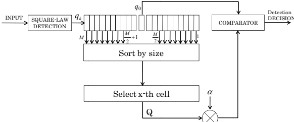
図 2. OS-CFAR の信号処理ブロック図
