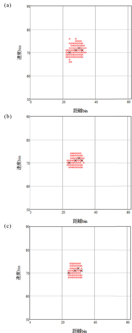
図 5. 合成帯域結果に対する OS-CFAR (1次元しきい値処理) による目標検知結果 ((a) \alpha=4 , (b) \alpha=8 , (c) \alpha=12 ) (黒: 目標設定値, 赤: 目標として検知された距離・速度ビン)
