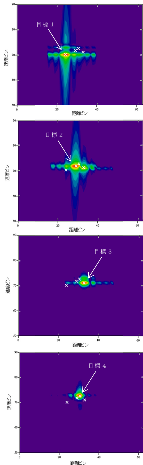
図 7. 目標の繰り返し減算による目標の自動検知結果 ((a) 目標 1, (b) 目標 2, (c) 目標 3, (d) 目標 4)
