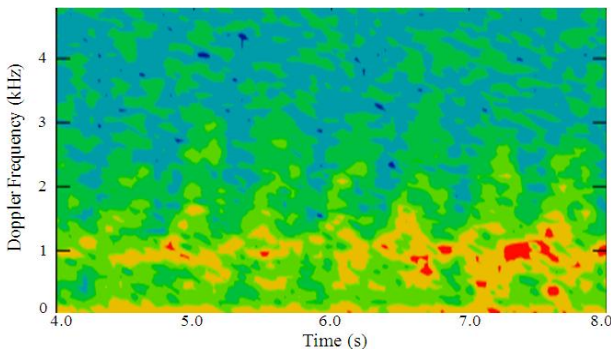
図 1 Doppler Frequency の時間変化 (人物歩行の例)
