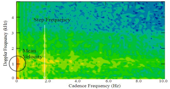
図 2 Cadence Frequency (同上データ)
